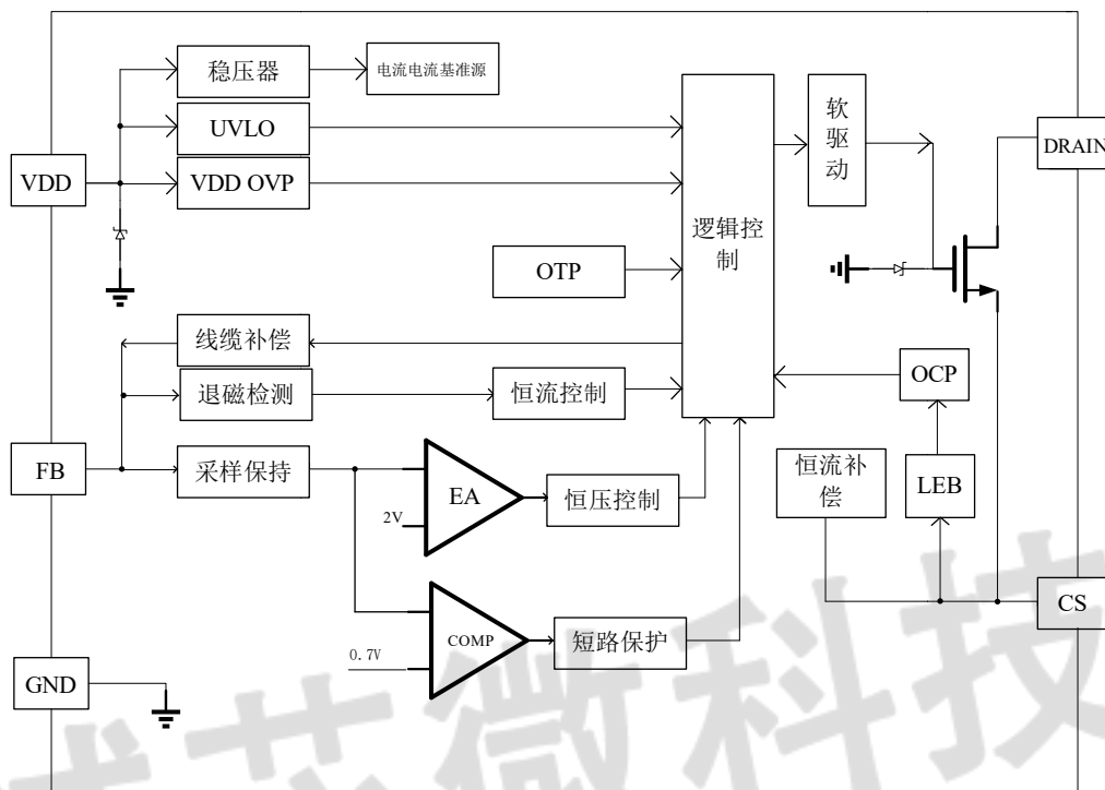
CX72XX系列 内部功能框图
